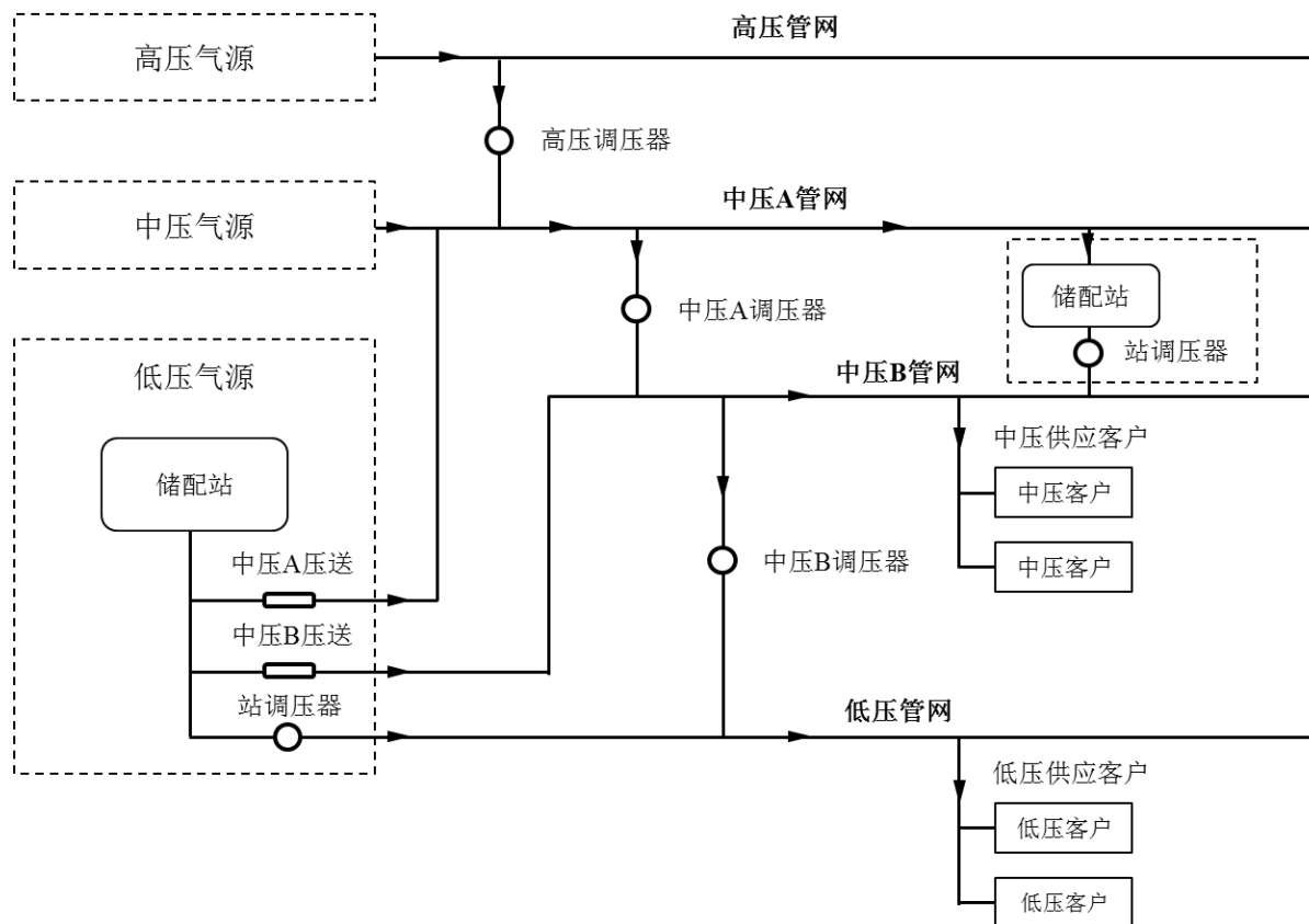
(2) 车用燃气销售业务流程图
