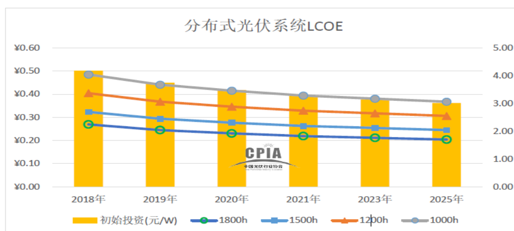
2018-2025 年分布式光伏系统不同等效利用小时数 LCOE 估算 (元/kWh)
