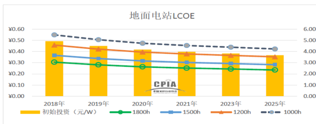
2018-2025 年光伏地面电站不同等效利用小时数 LCOE 估算 (元/kWh)
