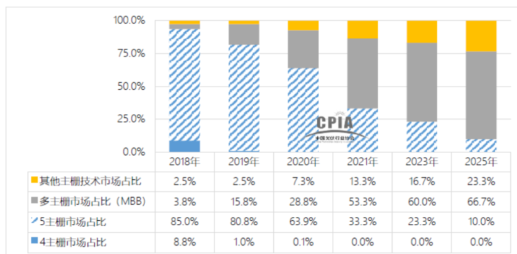
图 40 2018-2025 年各种主栅市场份额占比变化趋势
