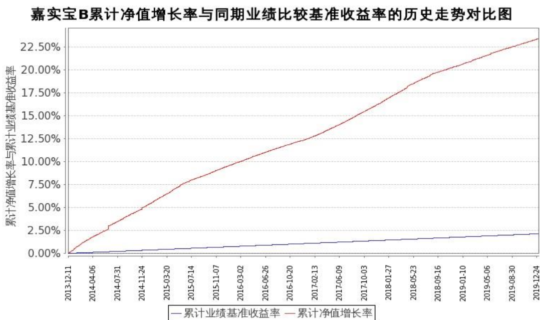
图 2：嘉实宝 B 基金份额累计净值收益率与同期业绩比较基准收益率的历史走势对比图 (2013 年 12 月 11 日至 2019 年 12 月 31 日)
