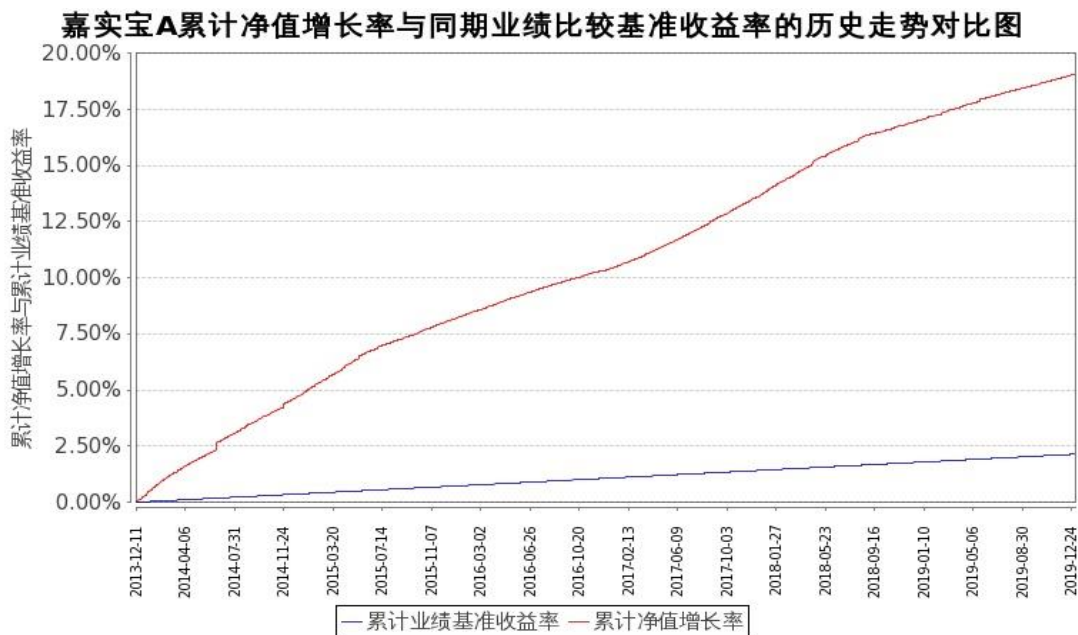
图 1：嘉实宝 A 基金份额累计净值收益率与同期业绩比较基准收益率的历史走势对比图 (2013 年 12 月 11 日至 2019 年 12 月 31 日)
