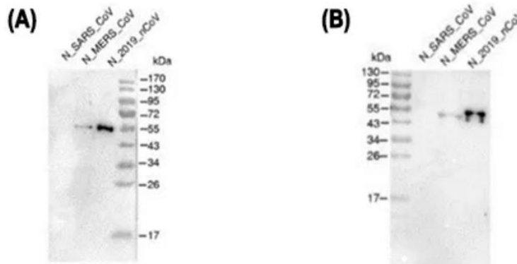
图解：使用SARS-CoV-2抗体对裂解液进行Western Blot分析。(A)单克隆(产品编号 A2060)；(B)多克隆(产品编号 A2061)
