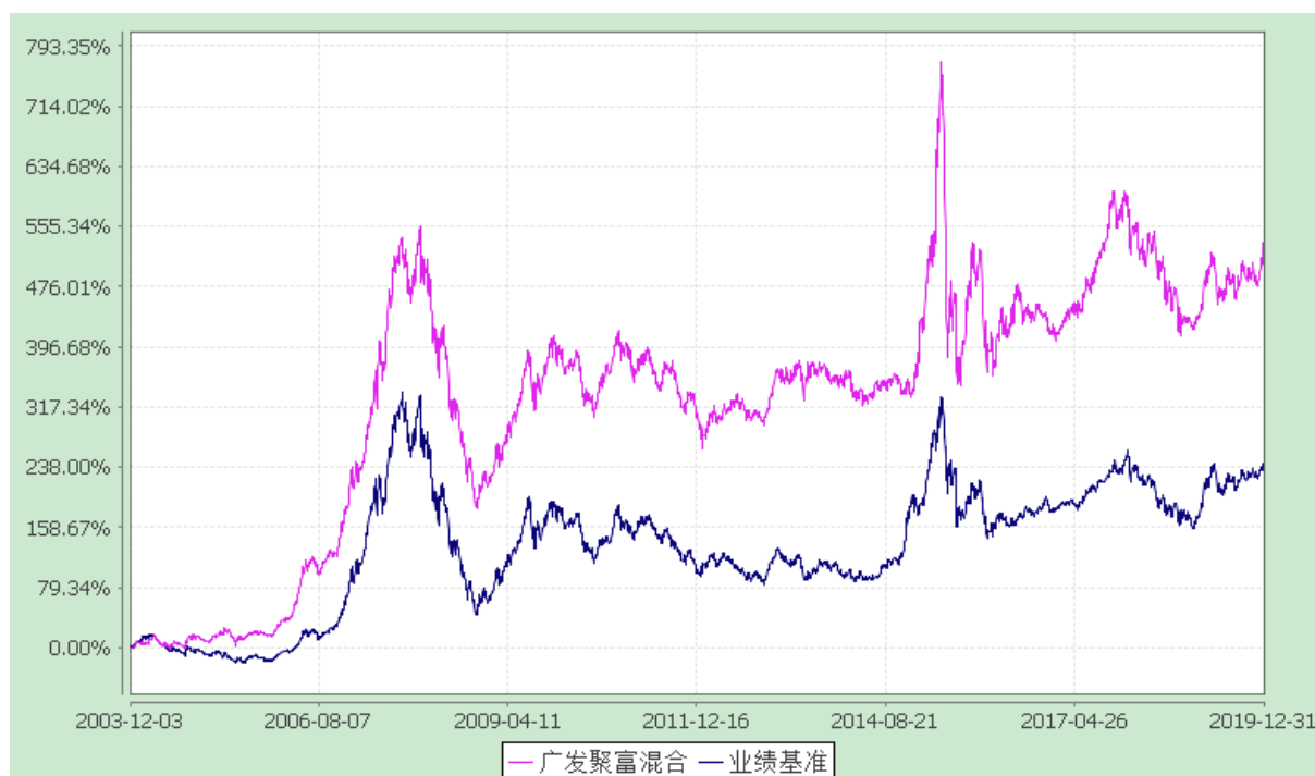
广发聚富开放式证券投资基金 份额累计净值增长率与业绩比较基准收益率的历史走势对比图 (2003 年 12 月 3 日至 2019 年 12 月 31 日)
