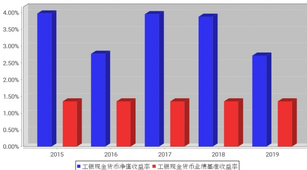
工银现金货币基金每年净值收益率与同期业绩比较基准收益率的对比图
