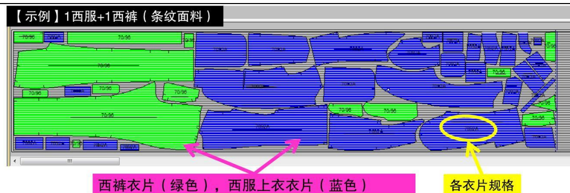
图表 6-15 自动制版生成衣片形状、排料图
