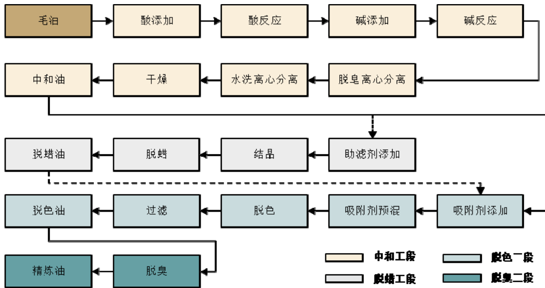
(3) 小包装食用油工艺流程图
