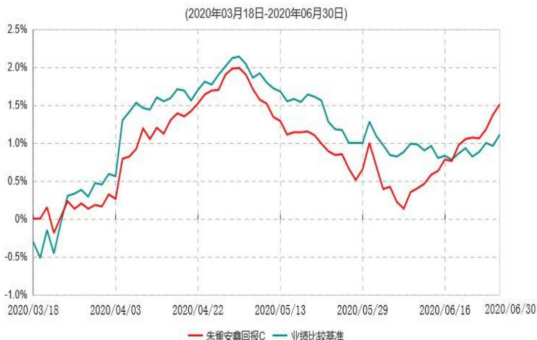
朱雀安鑫回报C累计净值增长率与业绩比较基准收益率历史走势对比图
