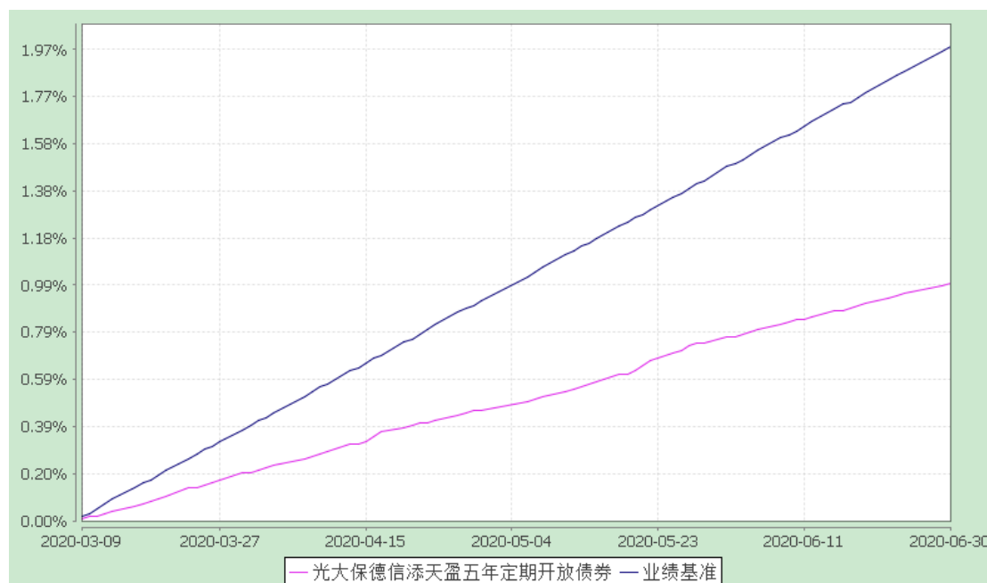
光大保德信添天盈五年定期开放债券型证券投资基金 累计净值增长率与业绩比较基准收益率历史走势对比图 (2020年3月9日至2020年6月30日)
