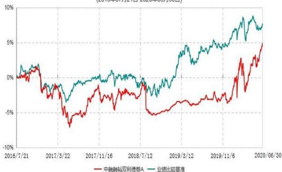
中融融裕双利债券A累计净值增长率与业绩比较基准收益率历史走势对比图
