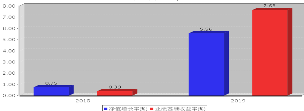
安信恒利增强债券A基金每年净值增长率与同期业绩比较基准收益率的对比图(2019年12月31日)
