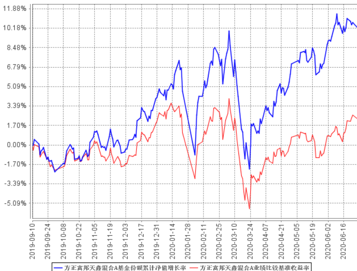
方正富邦天鑫混合A基金份额累计净值增长率与同期业绩比较基准收益率的历史走势对比图
