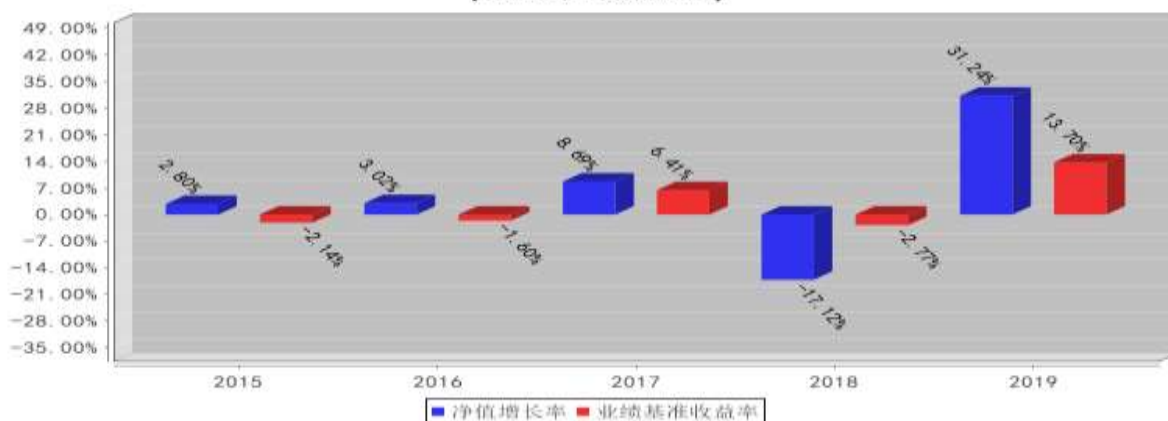
泰达宏利新起点混合A基金每年净值增长率与同期业绩比较基准收益率的对比图 (2019年12月31日)
