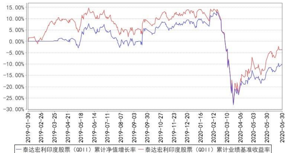
泰达宏利印度股票（QDII）累计净值增长率与同期业绩比较基准收益率的历史走势对比图
