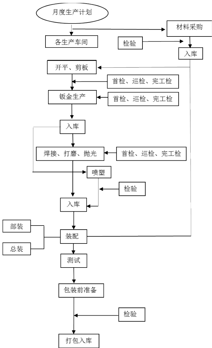
集成灶生产工艺流程图
