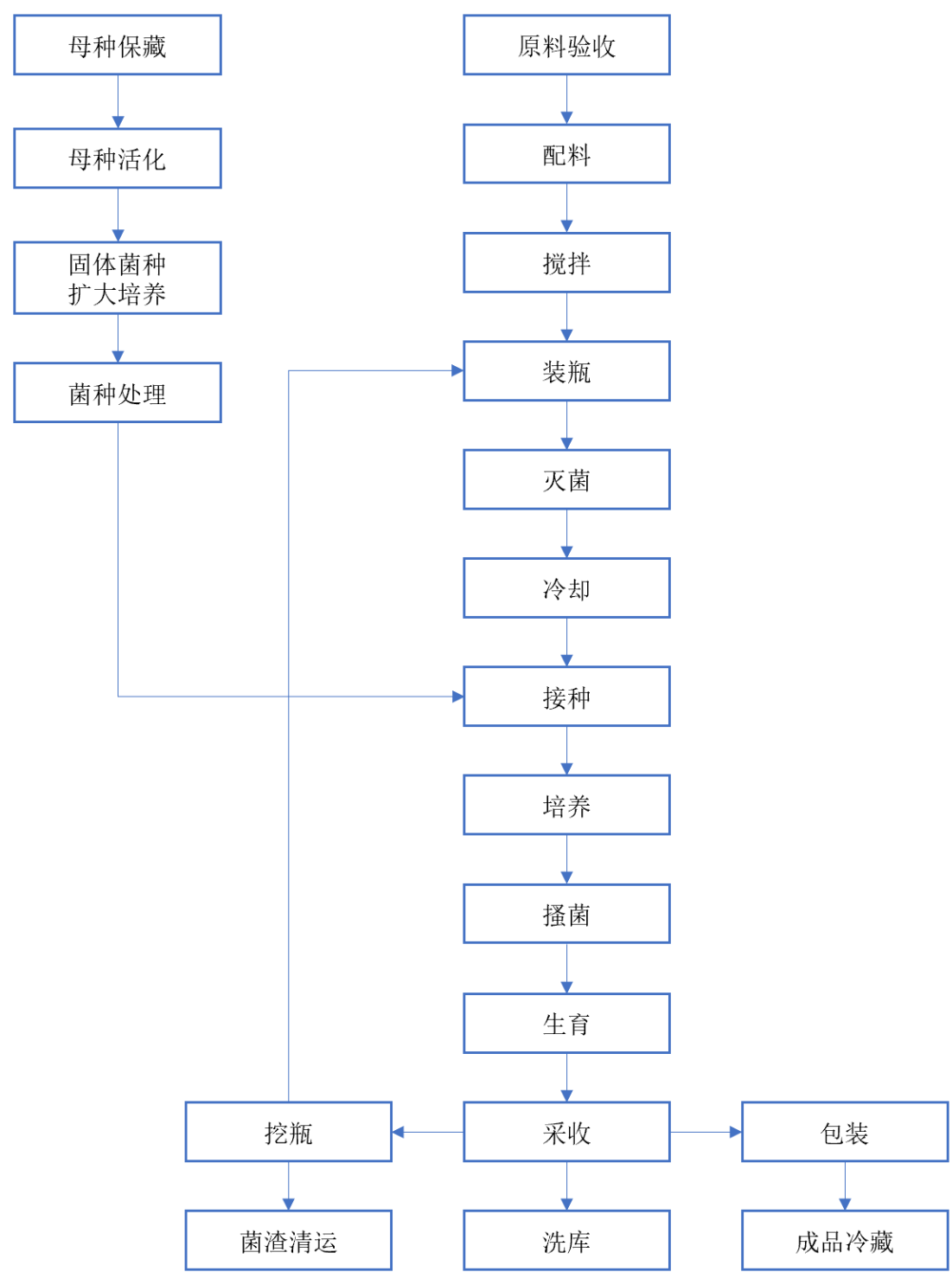
真姬菇（蟹味菇、白玉菇）工厂化生产的主要工艺流程描述如下表：
