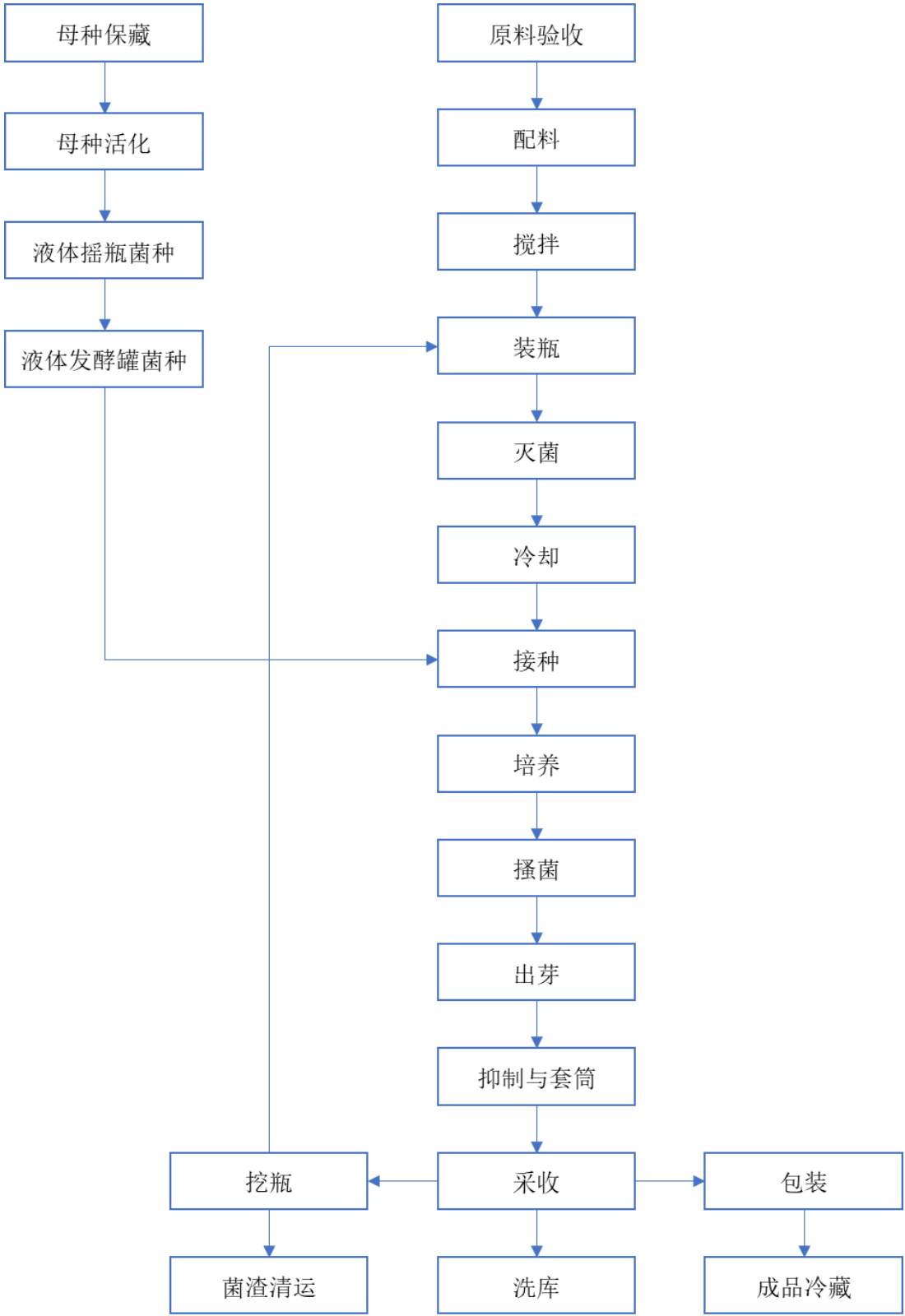
金针菇工厂化生产的主要工艺流程描述如下表：
