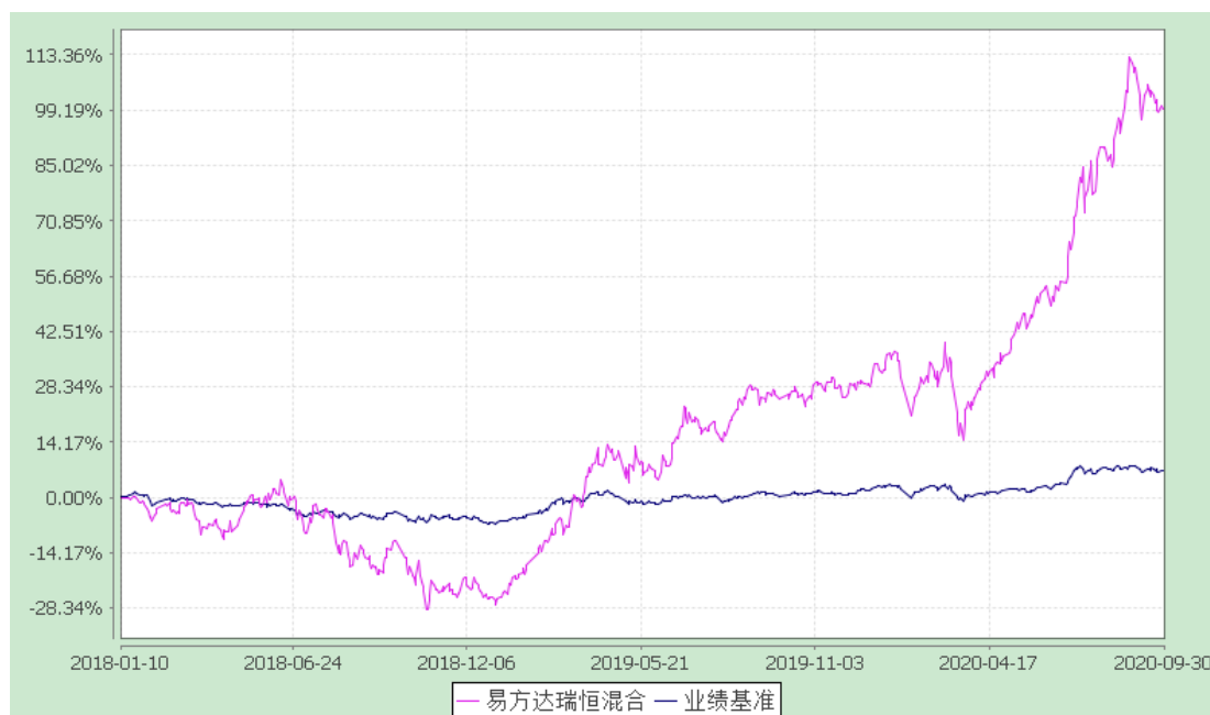
易方达瑞恒灵活配置混合型证券投资基金 累计净值增长率与业绩比较基准收益率的历史走势对比图 (2018 年 1 月 10 日至 2020 年 9 月 30 日)
