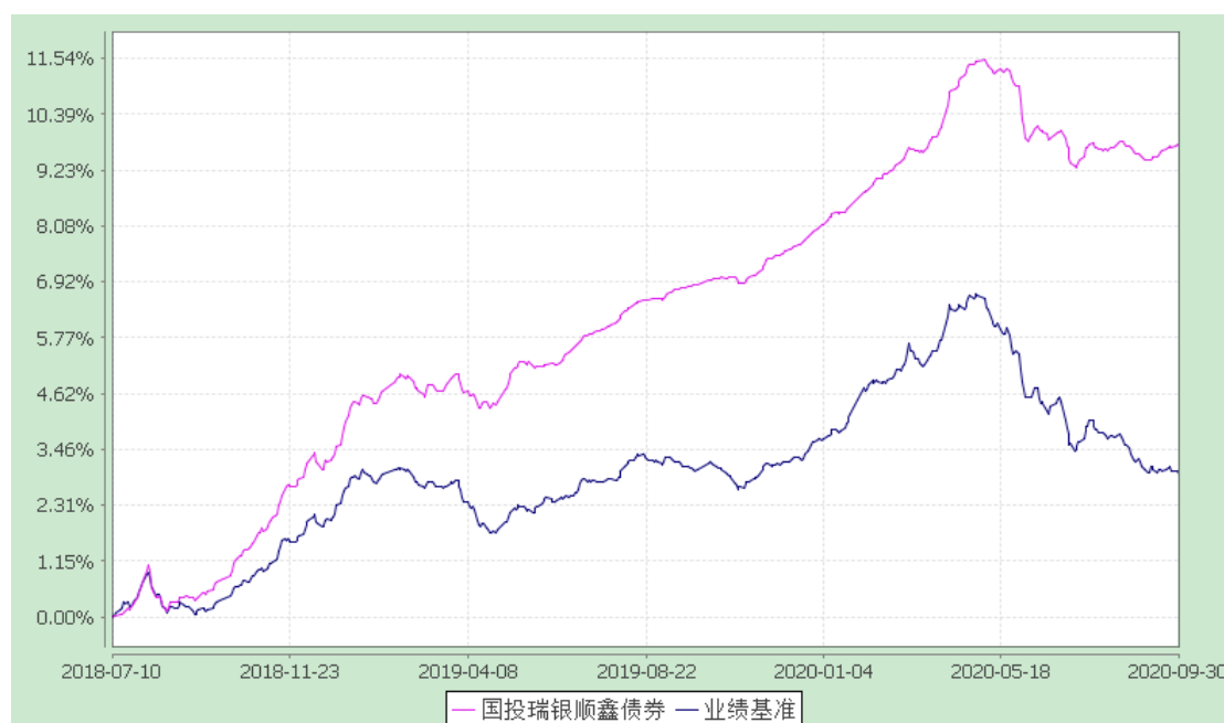
国投瑞银顺鑫定期开放债券型发起式证券投资基金 累计净值增长率与业绩比较基准收益率历史走势对比图 (2018 年 7 月 10 日至 2020 年 9 月 30 日)
