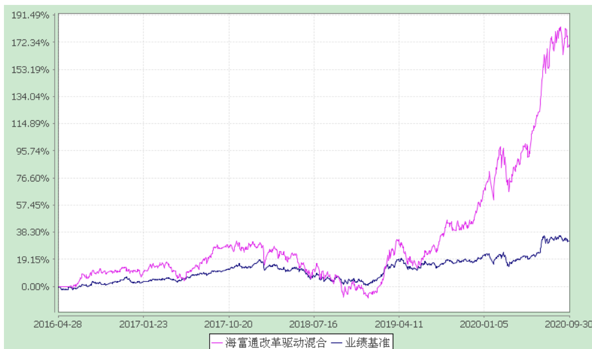
海富通改革驱动灵活配置混合型证券投资基金 份额累计净值增长率与业绩比较基准收益率历史走势对比图 (2016 年 4 月 28 日至 2020 年 9 月 30 日)
