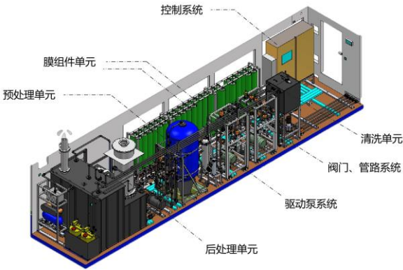
膜分离装备构造图
