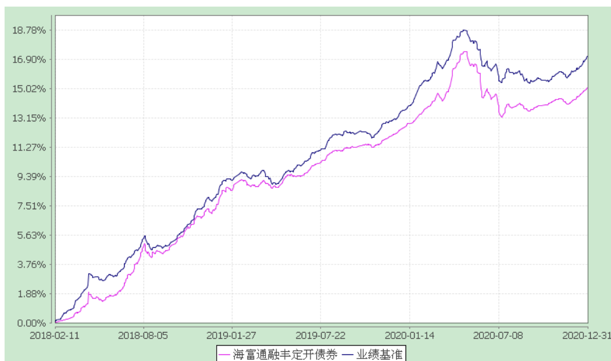
份额累计净值增长率与业绩比较基准收益率历史走势对比图 (2018 年 2 月 11 日至 2020 年 12 月 31 日)
