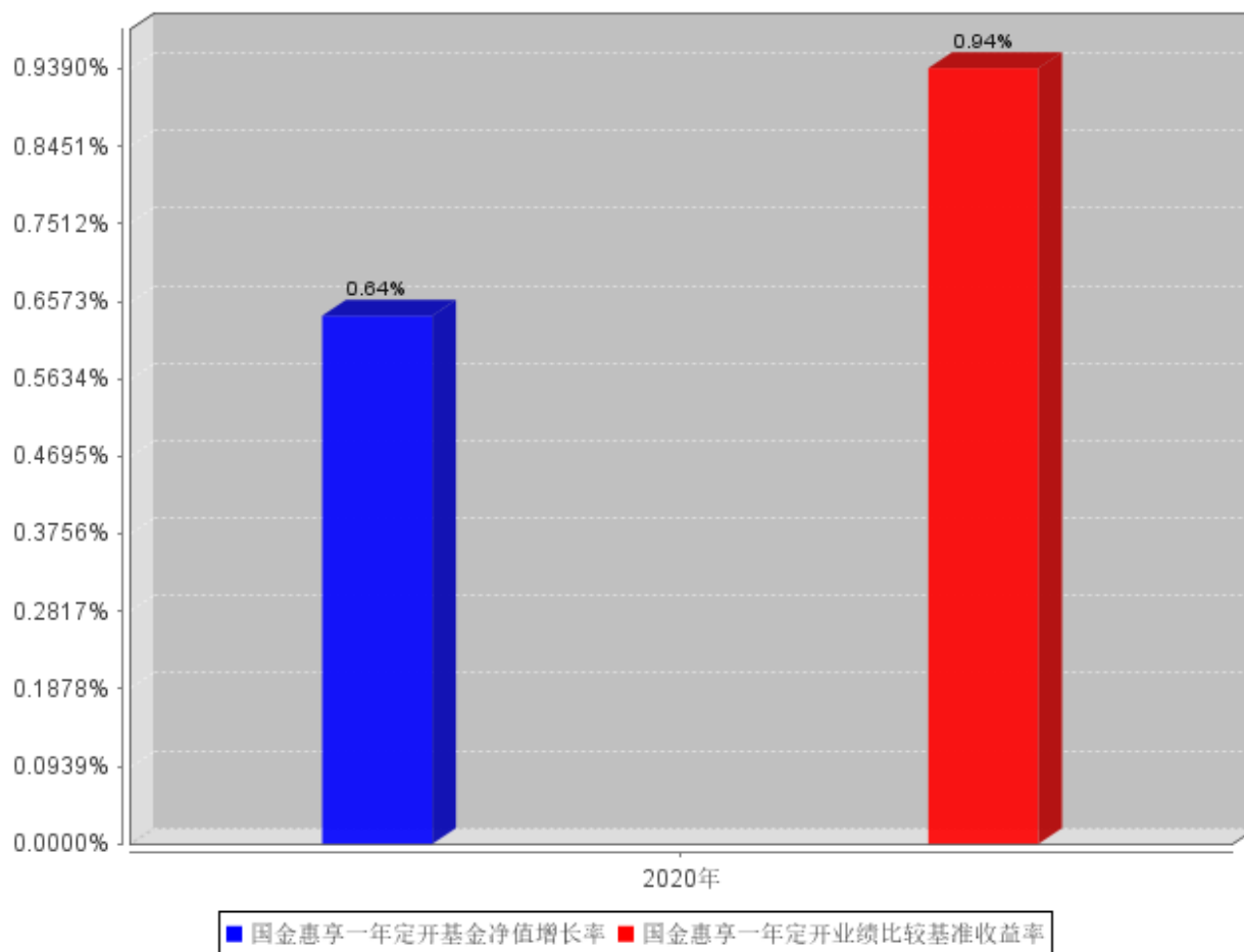
国金惠享一年定开自基金合同生效以来基金每年净值增长率及其与同期业绩比较基准收益率的对比图
