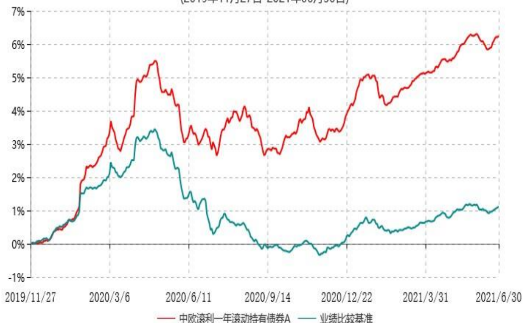
中欧滚利一年滚动持有债券A累计净值增长率与业绩比较基准收益率历史走势对比图 (2019年11月27日-2021年06月30日)
