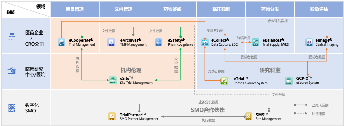
图：临床研究及药物警戒领域主要 SaaS 产品连接示意图
