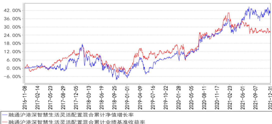
融通沪港深智慧生活灵活配置混合累计净值增长率与同期业绩比较基准收益率的历史走势对比图
