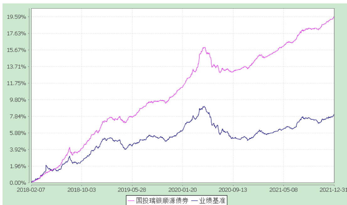
国投瑞银顺源 6 个月定期开放债券型证券投资基金 累计净值增长率与业绩比较基准收益率历史走势对比图 (2018 年 2 月 7 日至 2021 年 12 月 31 日)
