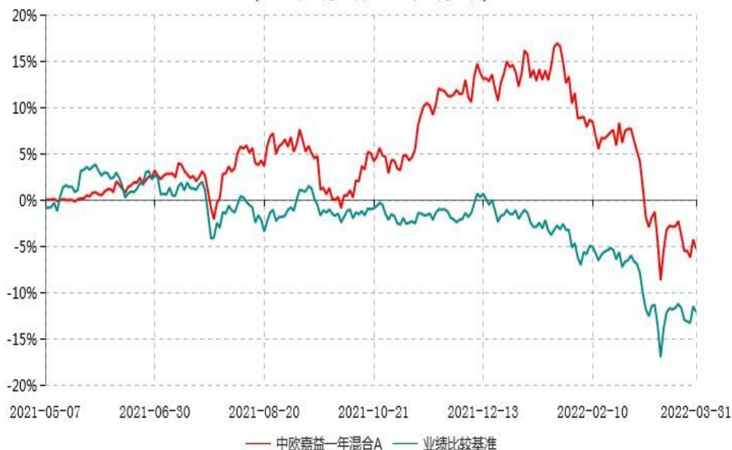
中欧嘉益一年混合A累计净值增长率与业绩比较基准收益率历史走势对比图 (2021年05月07日-2022年03月31日)
