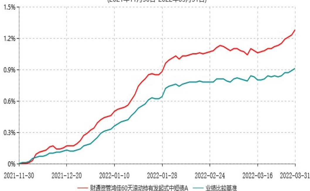
财通资管鸿佳60天滚动持有发起式中短债A累计净值增长率与业绩比较基准收益率历史走势对比图
