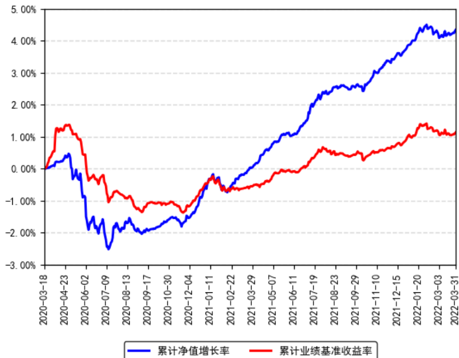
南方乐元中短利率债A累计净值增长率与同期业绩比较基准收益率的历史走势对比图
