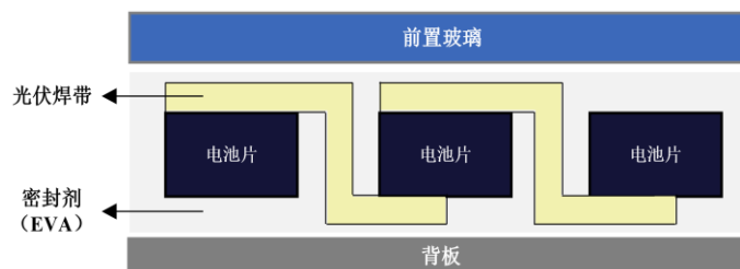
光伏焊带工作原理
