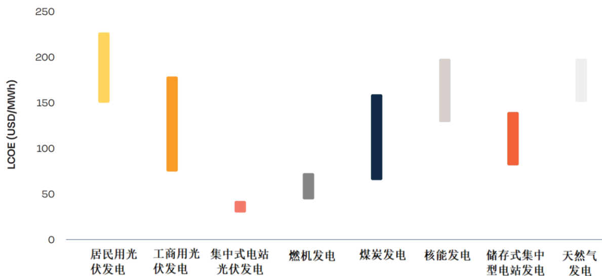
2020 年各类型能源发电平均成本（单位：美元/MWh）
