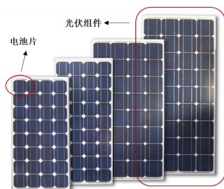
电池片与光伏组件
