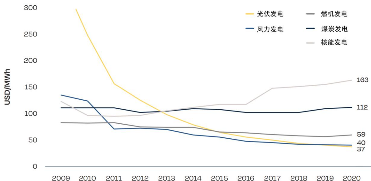
2009-2020 年各类能源发电平均成本变化趋势
