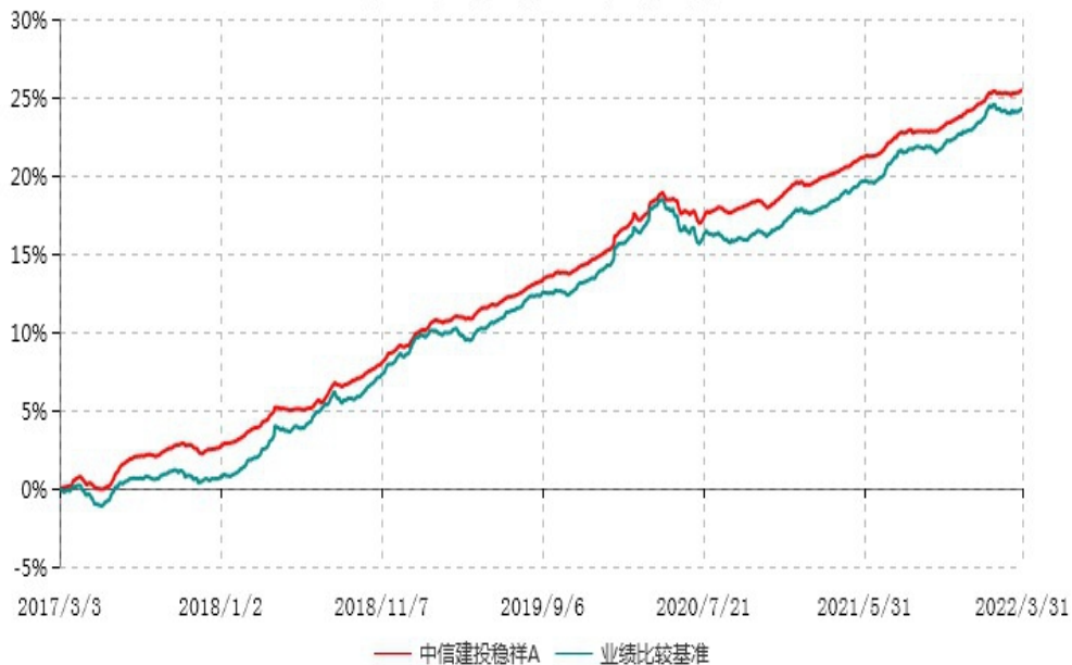
中信建投稳祥A累计净值增长率与业绩比较基准收益率历史走势对比图 (2017年03月03日-2022年03月31日)
