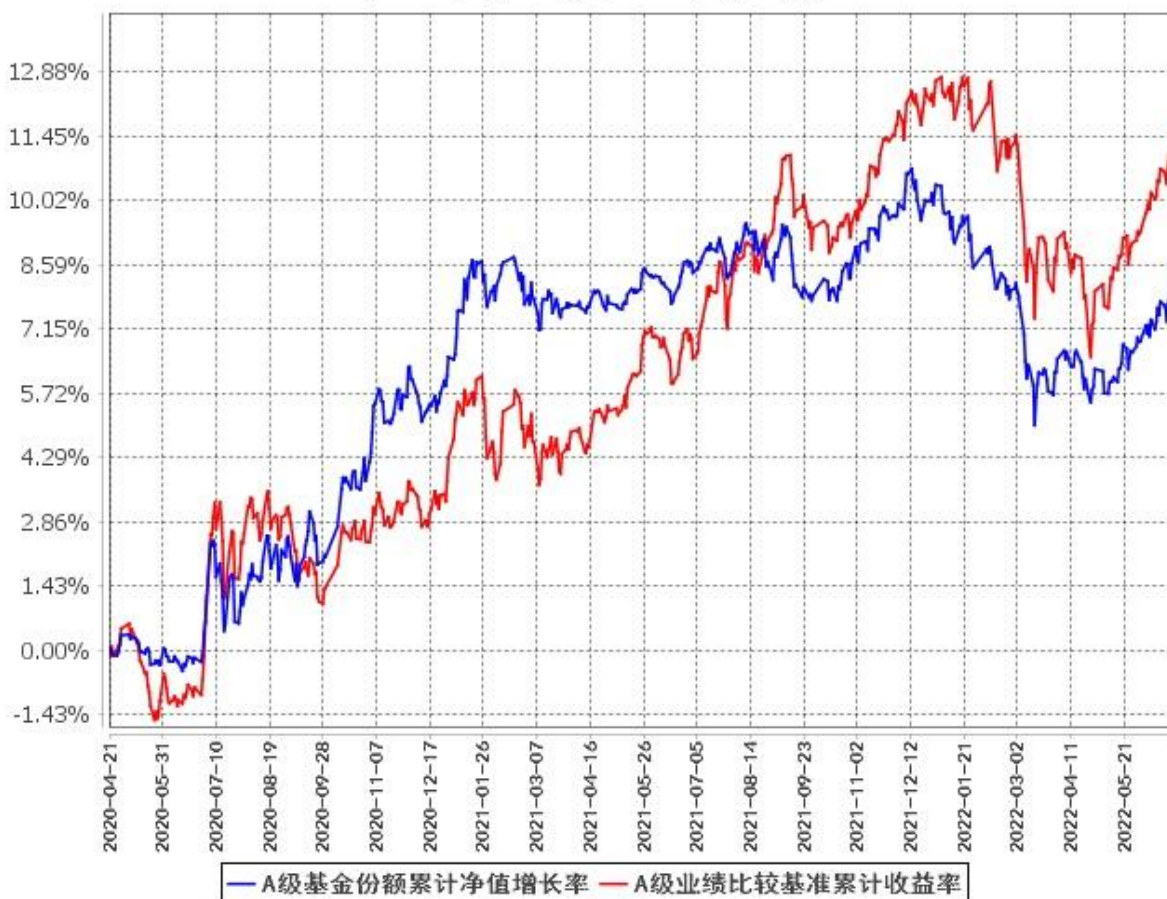
A级基金份额累计净值增长率与同期业绩比较基准收益率的历史走势对比图 (2020年4月21日至2022年6月30日)
