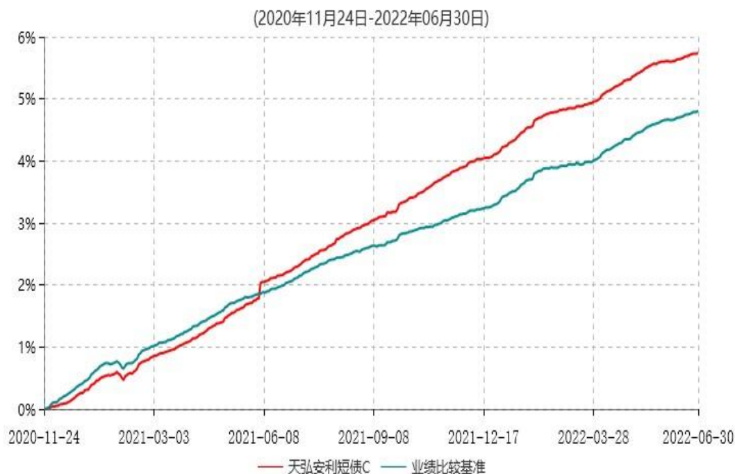
天弘安利短债C累计净值增长率与业绩比较基准收益率历史走势对比图
