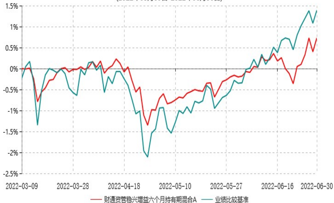
财通资管稳兴增益六个月持有期混合A累计净值增长率与业绩比较基准收益率历史走势对比图 (2022年03月09日-2022年06月30日)
