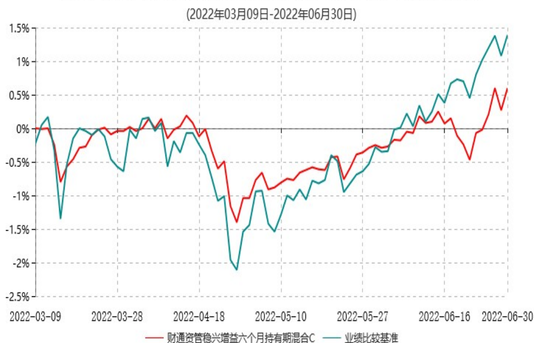
财通资管稳兴增益六个月持有期混合C累计净值增长率与业绩比较基准收益率历史走势对比图
