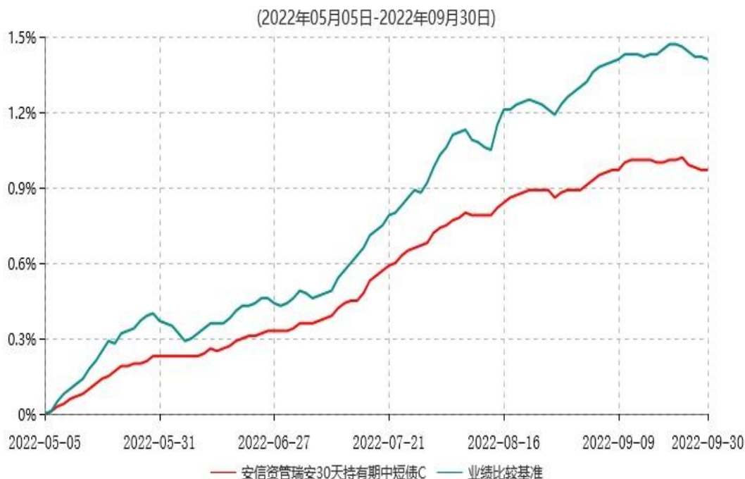
安信资管瑞安30天持有期中短债C累计净值增长率与业绩比较基准收益率历史走势对比图
