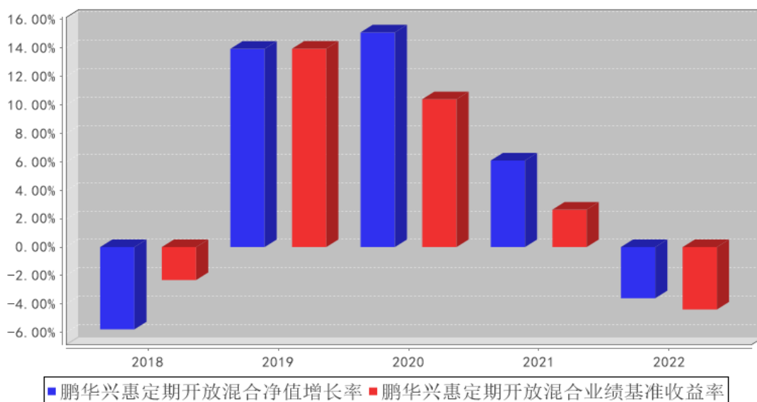
鹏华兴惠定期开放混合基金每年净值增长率与同期业绩比较基准收益率的对比图
