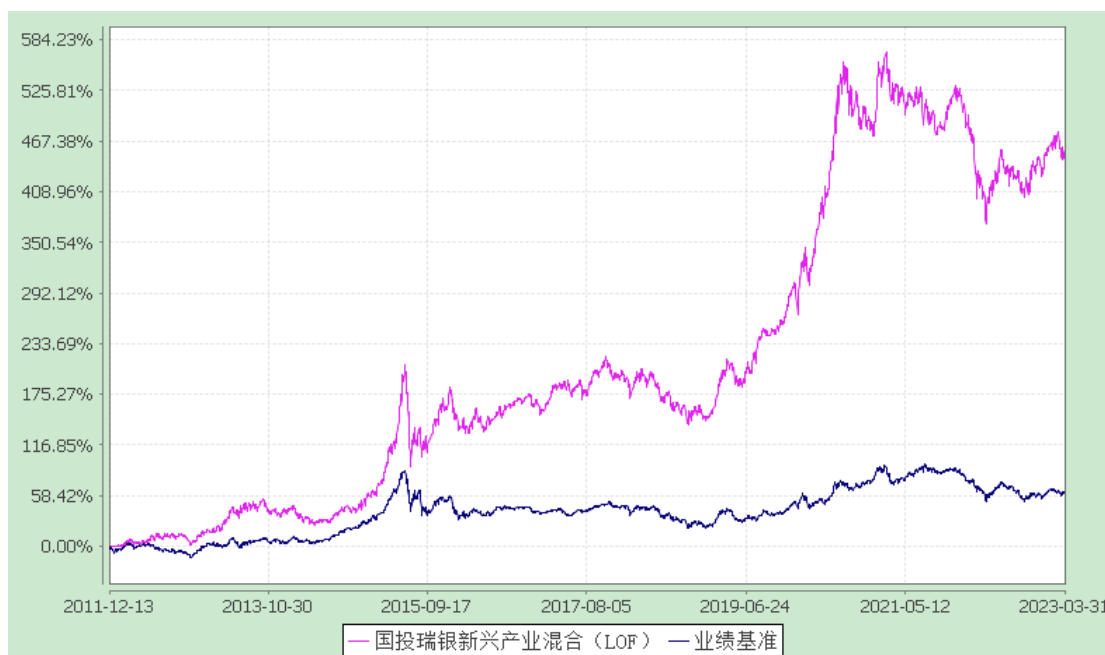
国投瑞银新兴产业混合型证券投资基金(LOF) 累计净值增长率与业绩比较基准收益率历史走势对比图 (2011 年 12 月 13 日至 2023 年 3 月 31 日)
