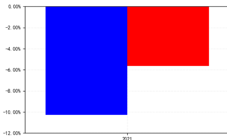
南方卓越优选3个月持有混合C每年净值增长率与同期业绩比较基准收益率的对比图（2021年12月31日）
