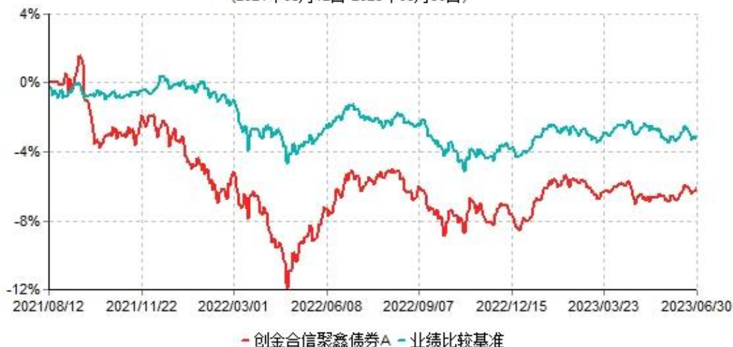
创金合信聚鑫债券A累计净值增长率与业绩比较基准收益率历史走势对比图 (2021年08月12日-2023年06月30日)
