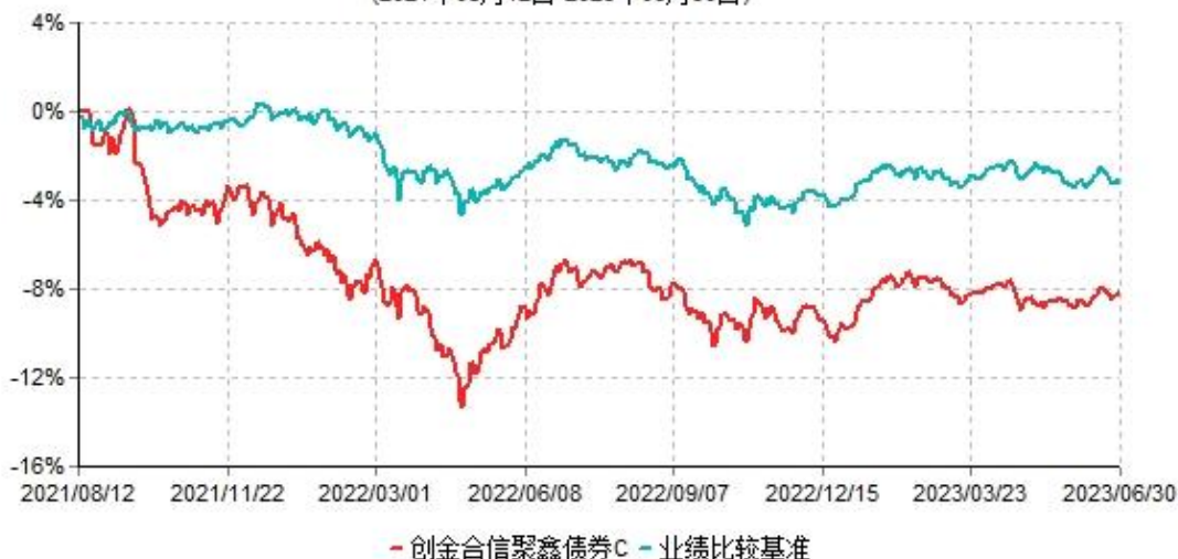
创金合信聚鑫债券C累计净值增长率与业绩比较基准收益率历史走势对比图 (2021年08月12日-2023年06月30日)
