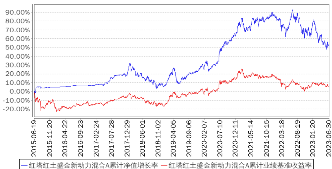
红塔红土盛金新动力混合A累计净值增长率与同期业绩比较基准收益率的历史走势对比图
