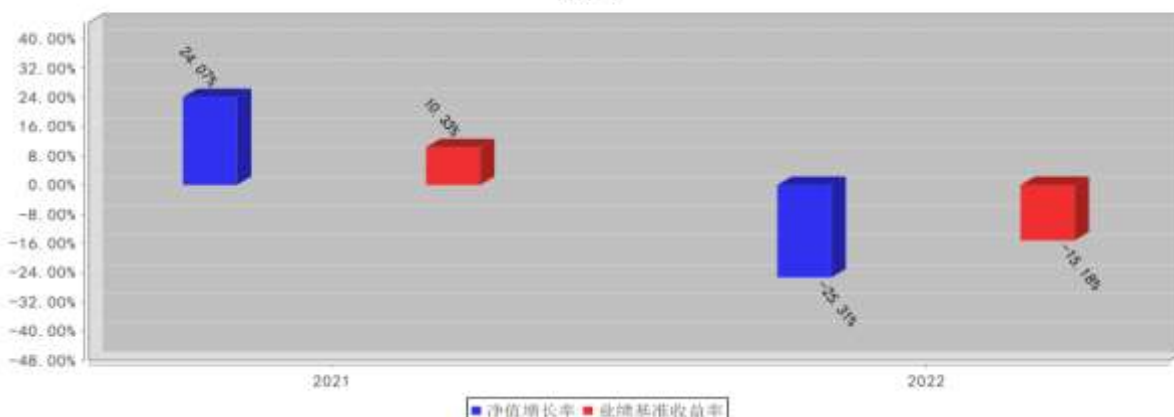
西部利得量化优选一年持有期混合A基金每年净值增长率与同期业绩比较基准收益率的对比图（2022年12月31日）
