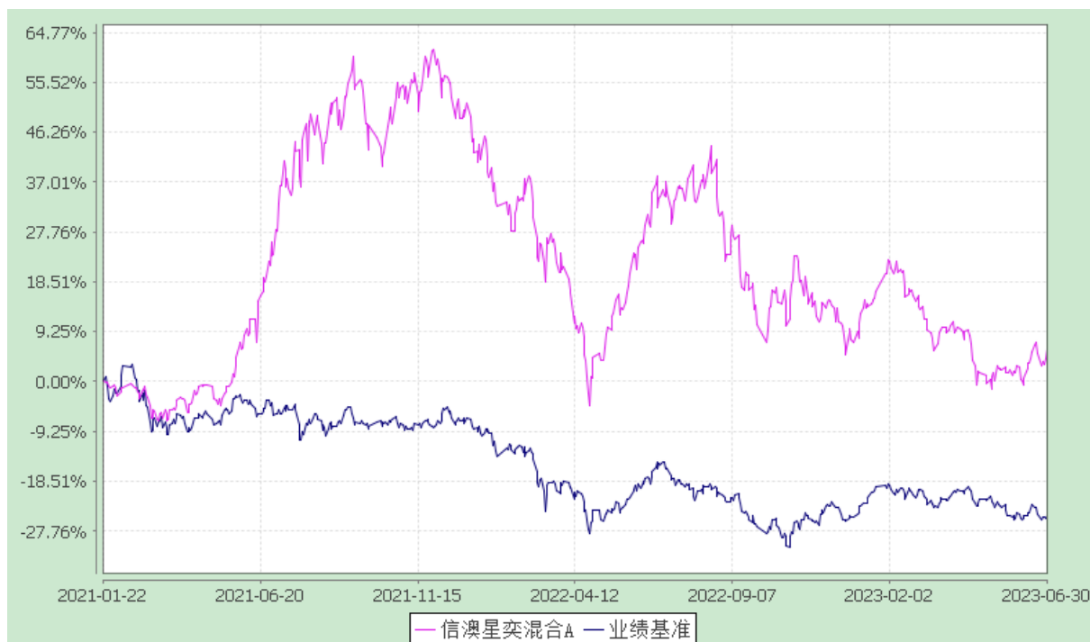
信澳星奕混合 C 累计净值增长率与业绩比较基准收益率的历史走势对比图 (2021 年 1 月 22 日至 2023 年 6 月 30 日)
