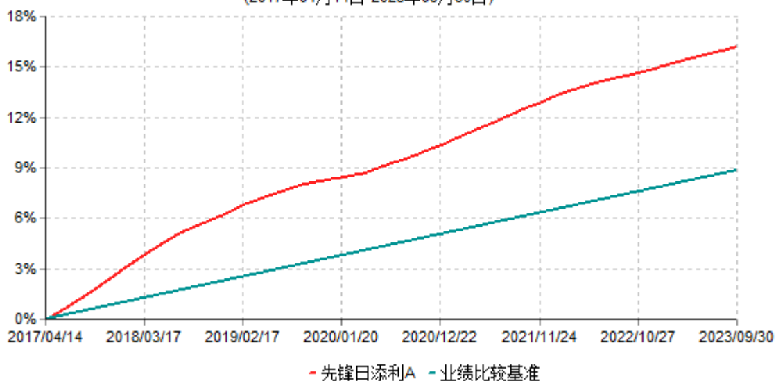
先锋日添利A累计净值收益率与业绩比较基准收益率历史走势对比图 (2017年04月14日-2023年09月30日)
