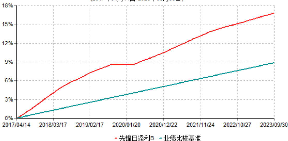
先锋日添利B累计净值收益率与业绩比较基准收益率历史走势对比图 (2017年04月14日-2023年09月30日)
