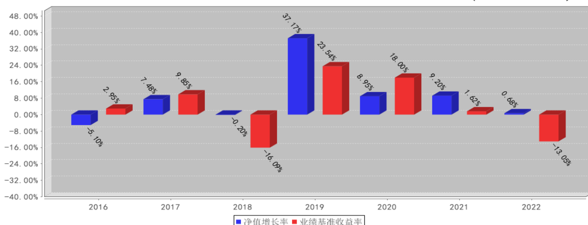
金信智能中国2025混合基金每年净值增长率与同期业绩比较基准收益率的对比图(2022年12月31日)
