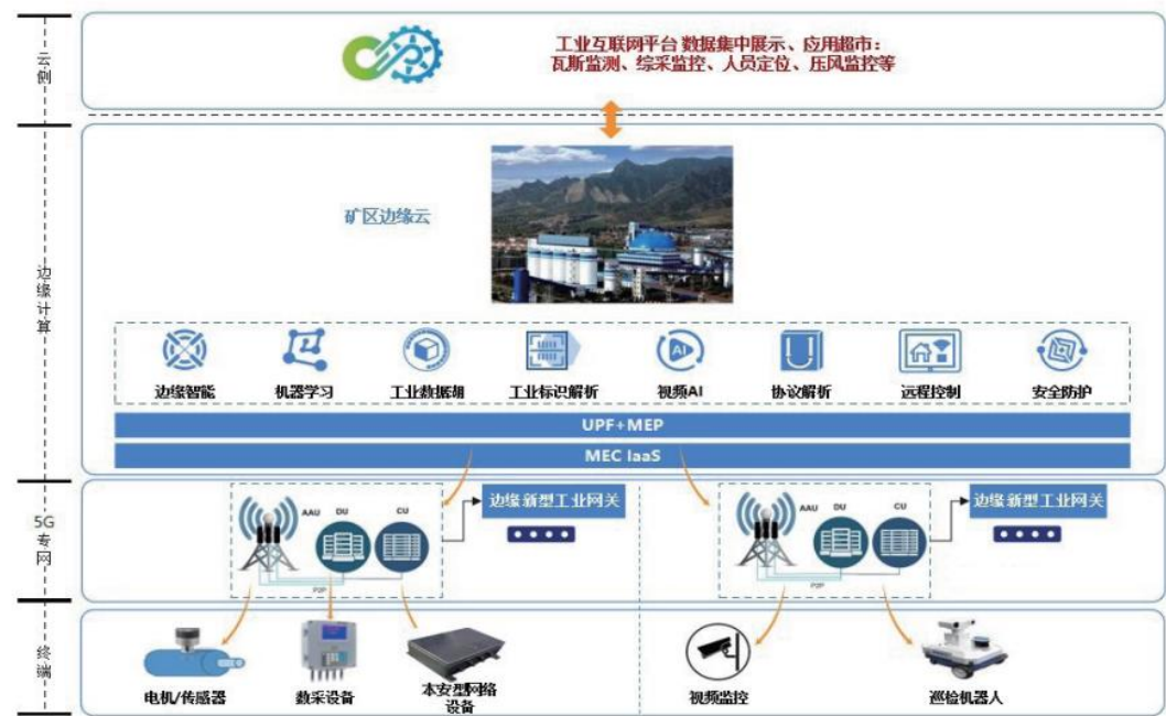
工业互联网云端、边端协同典型架构
