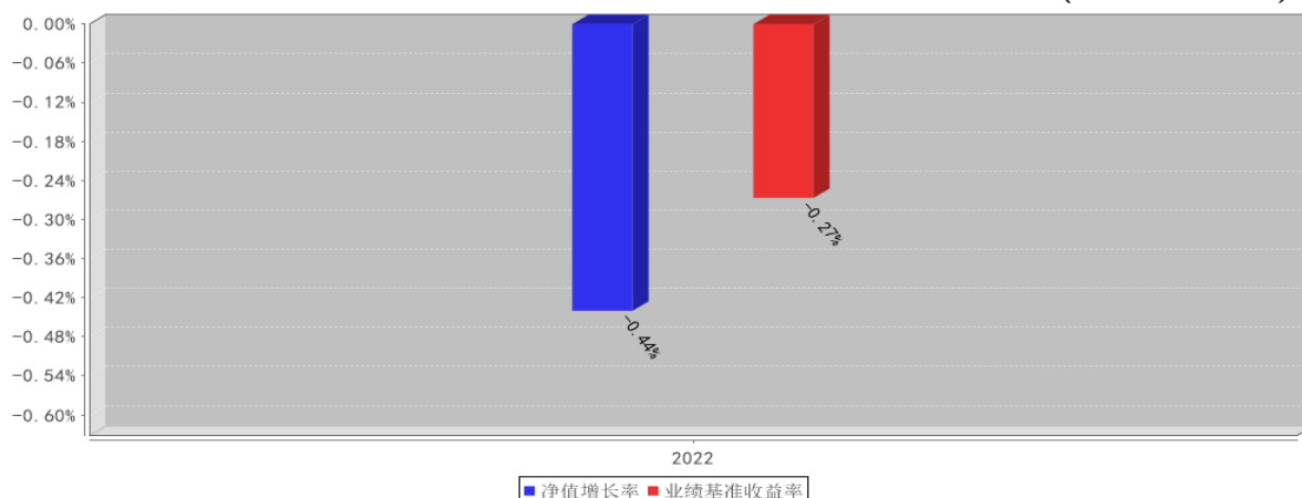
长信稳兴三个月定开债券C基金每年净值增长率与同期业绩比较基准收益率的对比图（2022年12月31日）
