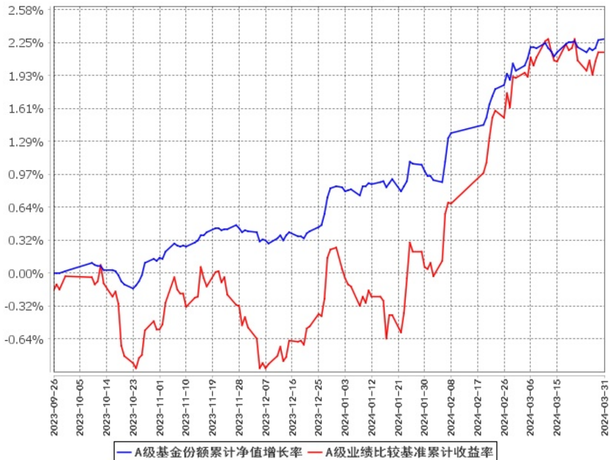
A级基金份额累计净值增长率与同期业绩比较基准收益率的历史走势对比图 (2023年9月26日至2024年3月31日)
