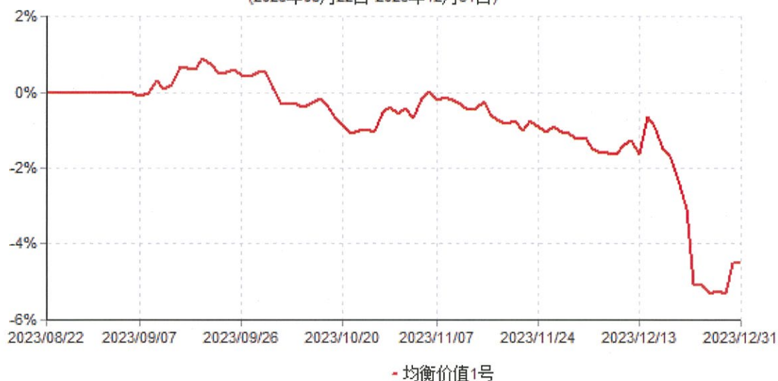
野村东方国际均衡价值1号集合资产管理计划累计净值增长率走势图 (2023年08月22日-2023年12月31日)
