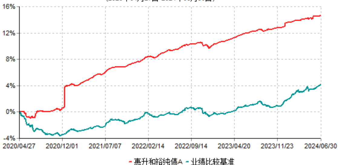
惠升和裕纯债A累计净值增长率与业绩比较基准收益率历史走势对比图 (2020年04月27日-2024年06月30日)
