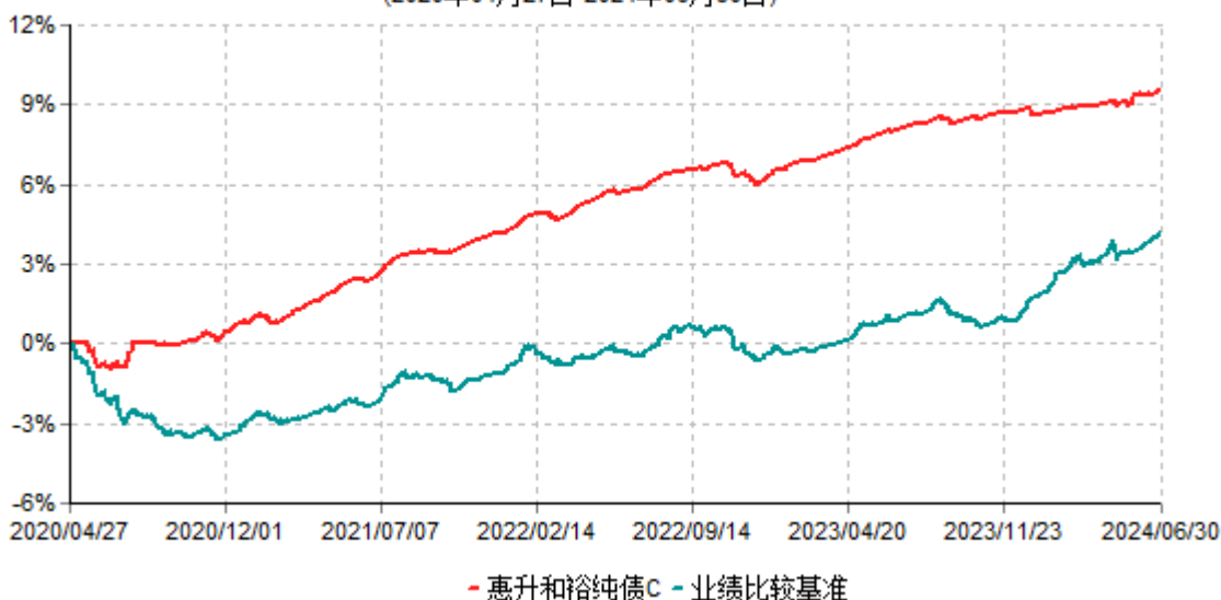
惠升和裕纯债C累计净值增长率与业绩比较基准收益率历史走势对比图 (2020年04月27日-2024年06月30日)
